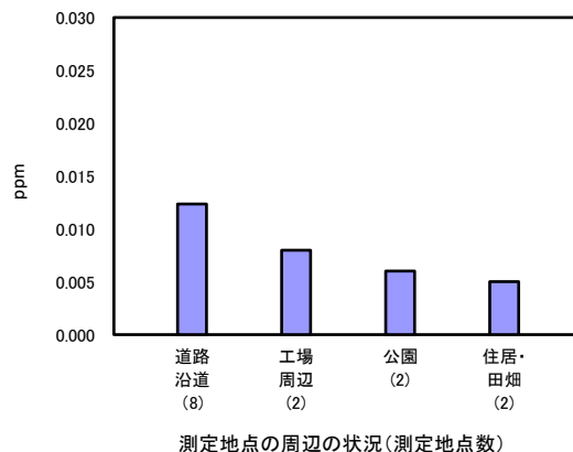
簡易測定による二酸化窒素の測定結果(令和元年度 年間結果)
