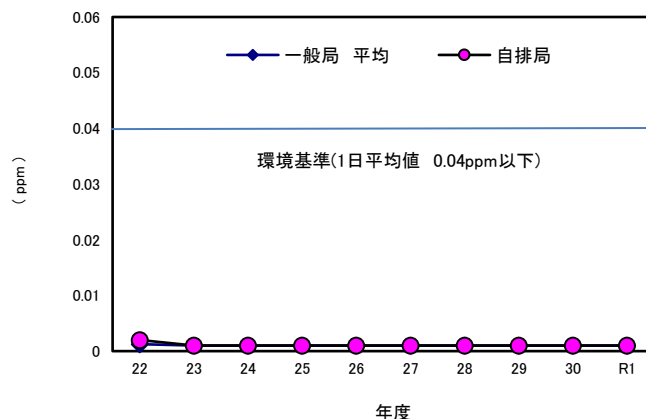
市内の二酸化硫黄経年変化(年間平均値)
