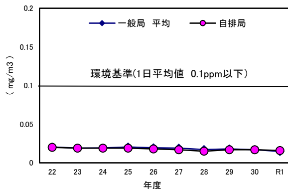
市内のSPM経年変化 (年間平均値)
